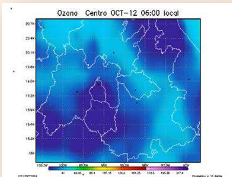
Modelos calidad del aire
