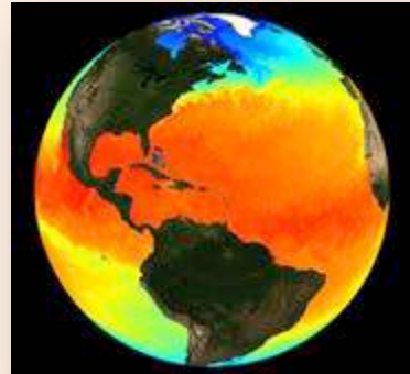
Temperatura del océano
