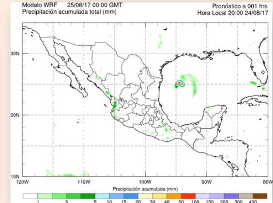
Precipitación: Huracán Harvey
